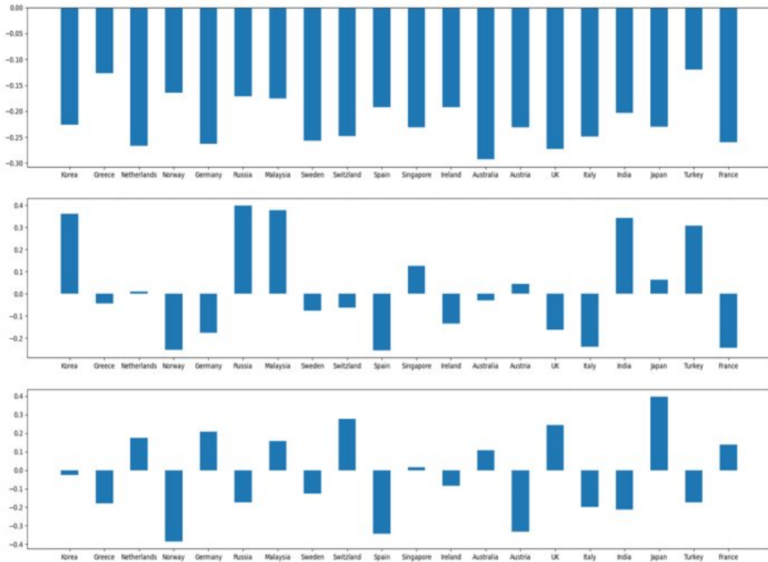
<그림 3> 국가별 시스템 리스크의 주성분 로딩값
