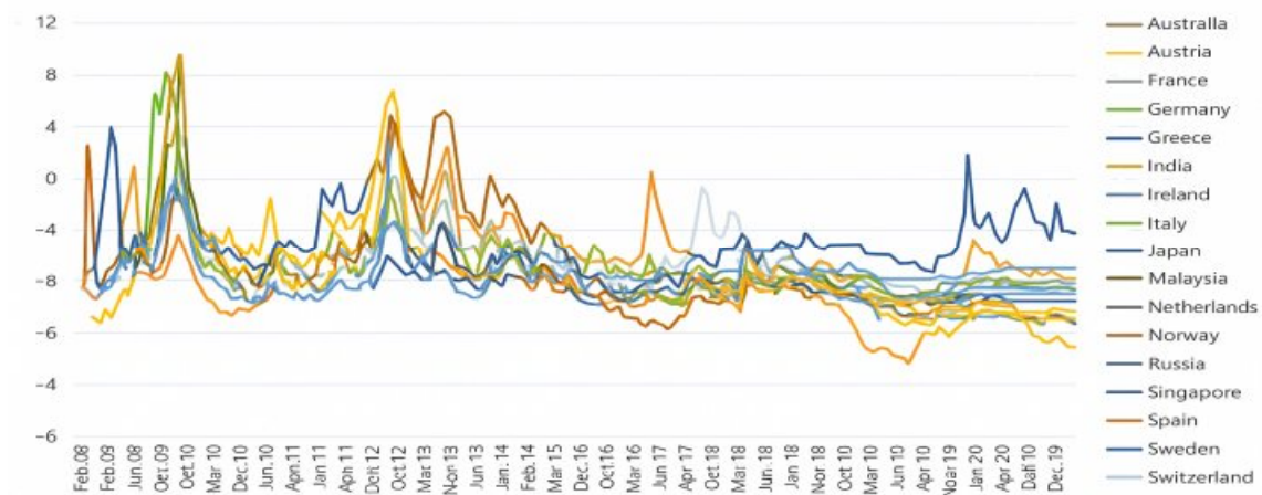
<그림 2> 국가별 시스템 리스크(PC1) 시계열
