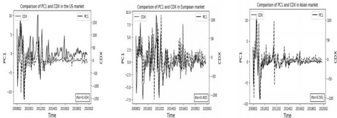
<그림1> PCA 접근법과 CDX 지수 비교
